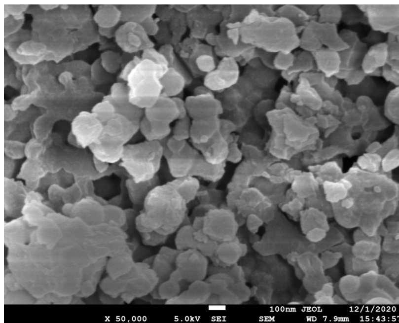
扫描电镜图
